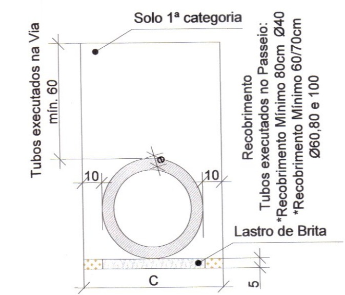
DIMENSÕES DAS VALAS PARA ASSENTAMENTO DOS TUBOS ESC.: 1/20
